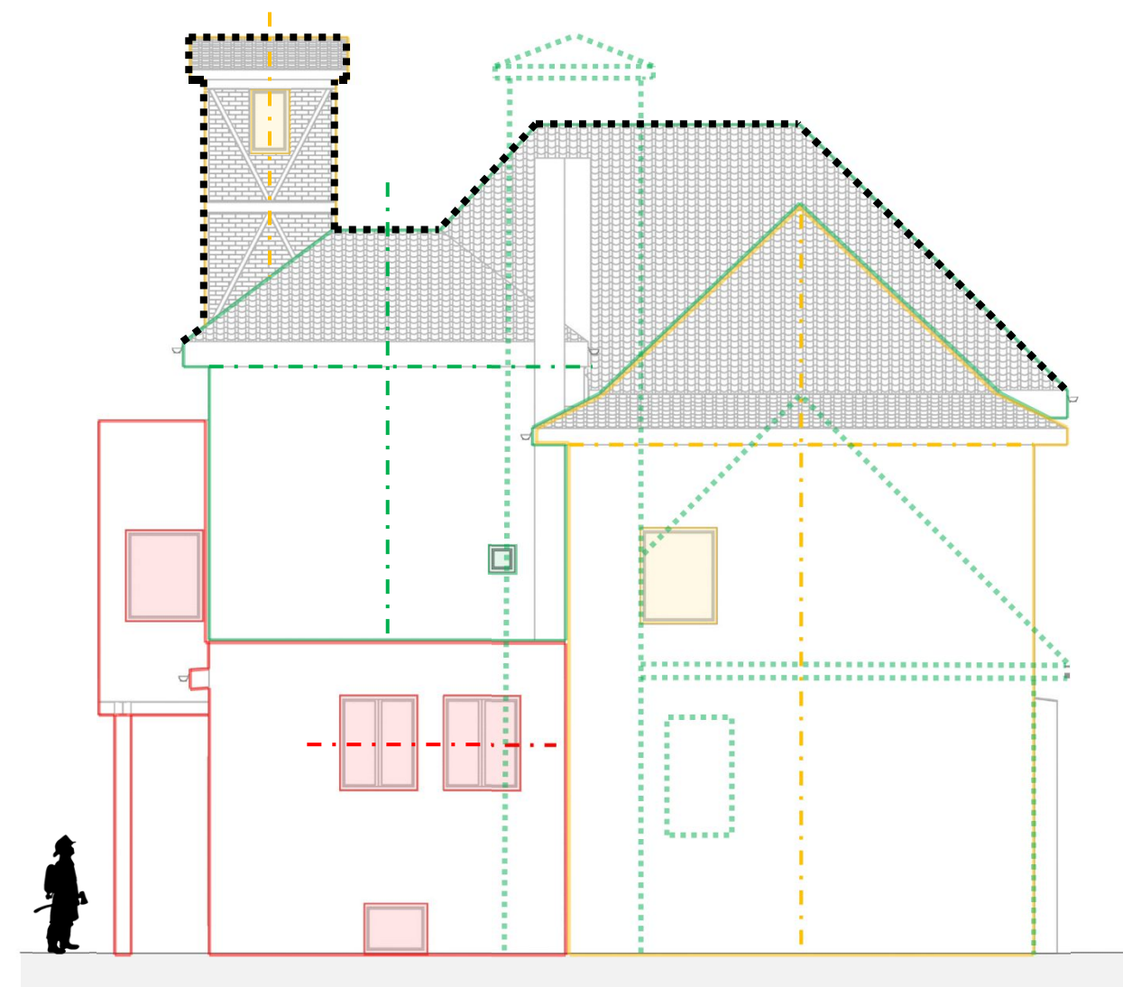
Jihovýchodní pohled
