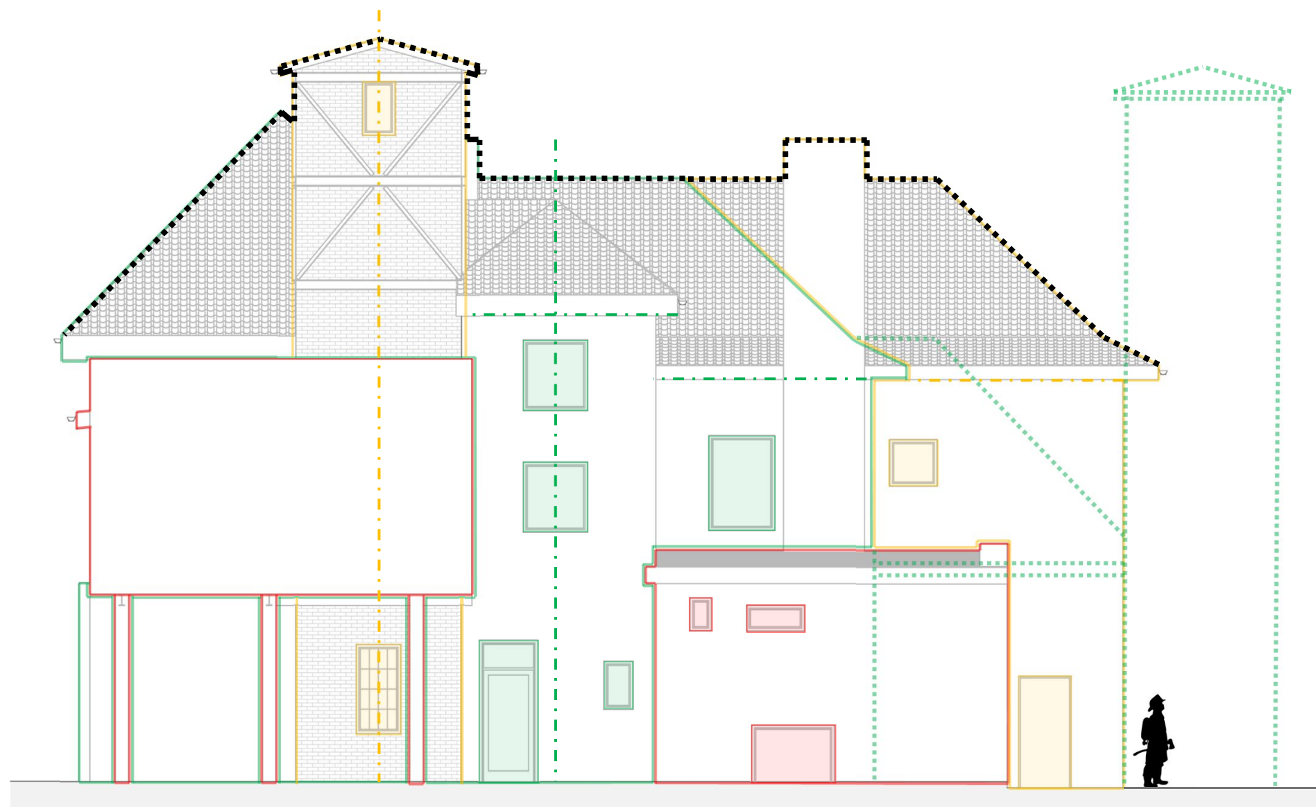
Jihozápadní pohled
