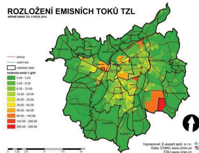
Obrázek č. 7 Rozložení emisních toků TZL, všechny skupiny zdrojů - roční průměr, rok 2010, Ostrava
